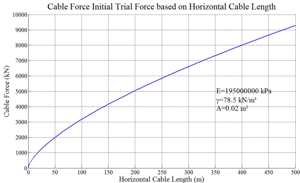
Figura 2 – Curva da estimativa inicial da força do cabo em função do comprimento em projeção horizontal do cabo para uma relação E_{eq}/E de 80% para o cabo com os dados fornecido no gráfico.
