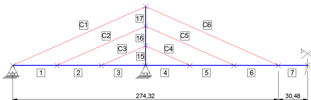
Figura 3 – Geometria da ponte estaiada com configuração em harpa com eixo de simetria e a numeração dos elementos finitos.
