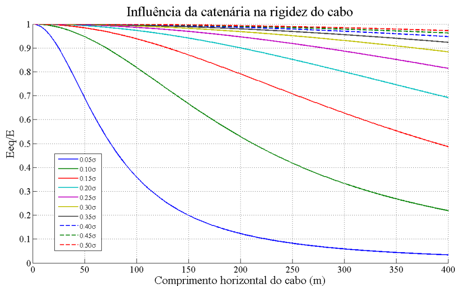
Figura 1 – Variação da razão entre módulo de Dischinger e módulo de elasticidade real em função do comprimento da projeção horizontal do cabo [Walther et al., 1988 - adaptado].
