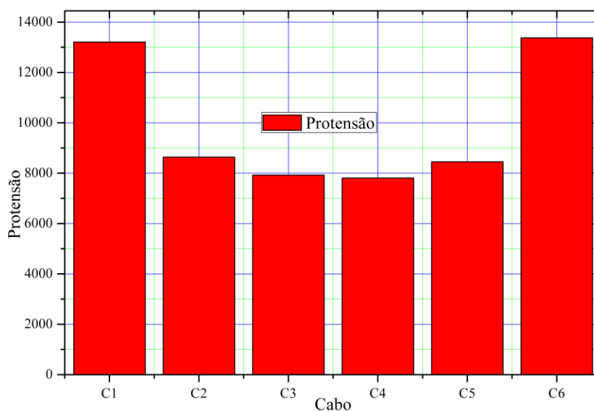
Figura 5 – Forças de protensão obtidas pelo método M.A.D.
