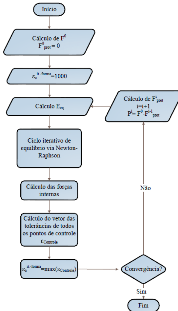
Figura 3 – Fluxograma do método M.A.D.
