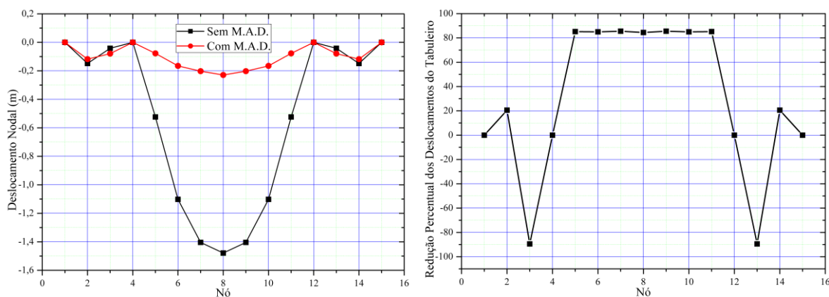
Figura 6 – Deslocamento vertical dos nós do tabuleiro (esquerda), e Redução percentual dos deslocamentos do tabuleiro (direita).
