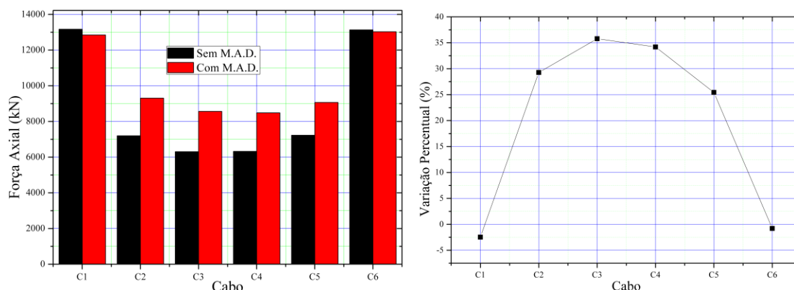
Figura 7 – Forças axiais nos cabos sem/com aplicação do método M.A.D. (esquerda), e Variação percentual das forças axiais nos cabos em relação a análise sem aplicação do método M.A.D. (direita).
