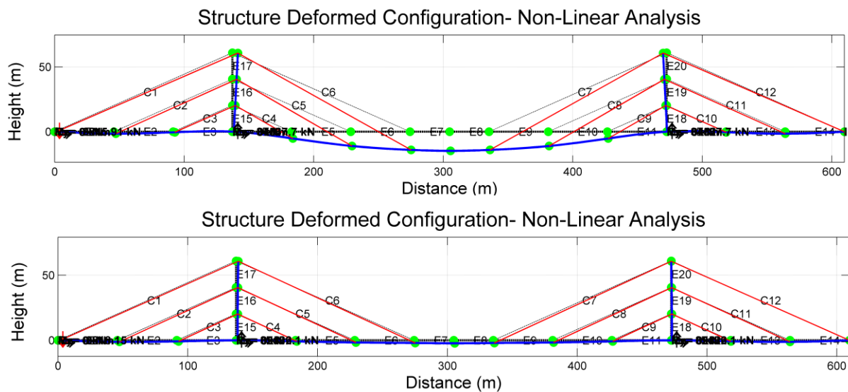
Figura 4 – Configurações deslocadas da estrutura com a análise não-linear (acima), e com análise não-linear com o método M.A.D. (abaixo).
