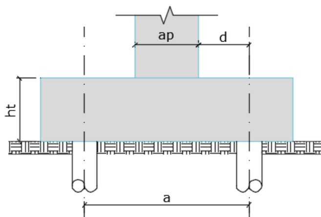
Figura 3 – Lajes apoiadas sobre estacas (CEB-70).
