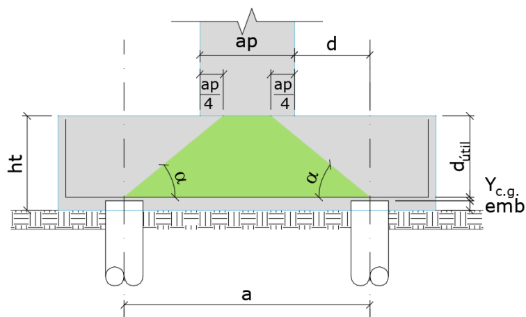
Figura 6 – Ângulo a ser efetivamente verificado.
