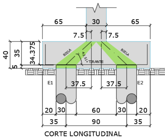
Figura 8 – Ângulo efetivo da biela.
