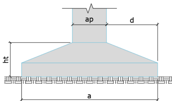
Figura 1.b – Lajes apoiadas sobre o solo (CEB-70).
