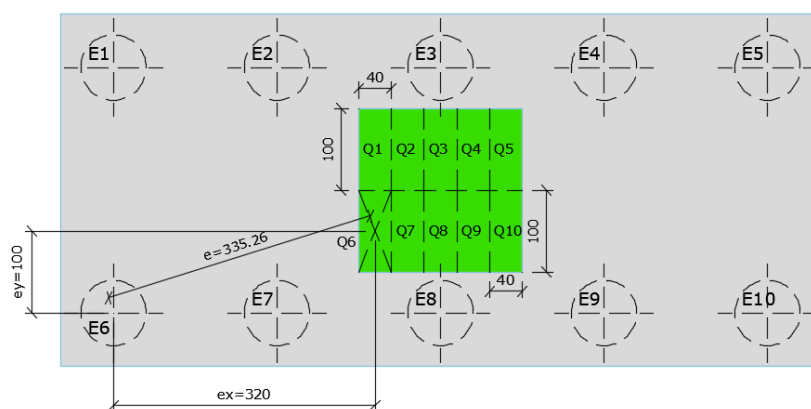
Figura 10 – Determinação da distância entre os C.G.'s.
