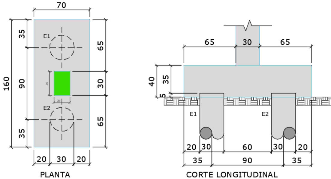
Figura 7 – Geometria do bloco de 2 estacas.
