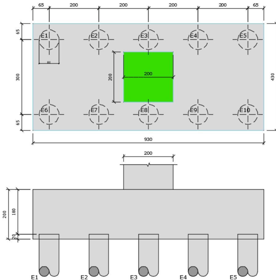
Figura 9 – Geometria do bloco de 10 estacas.
