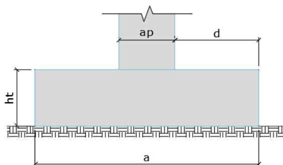
Figura 1.a – Lajes apoiadas sobre o solo (CEB-70).
