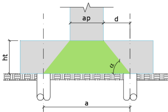
Figura 4 – Ângulo a ser verificado nos blocos (CEB-70).
