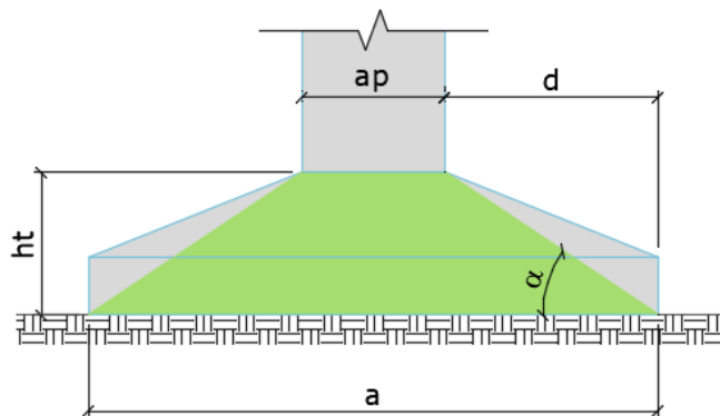
Figura 2 – Ângulo a ser verificado nas sapatas (CEB-70).
